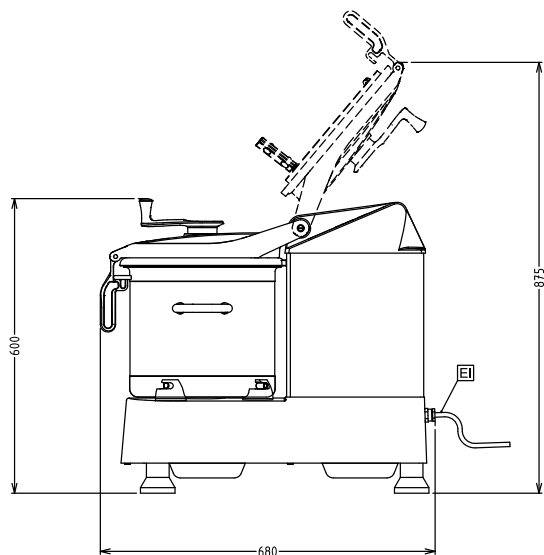
Oldalnézet
